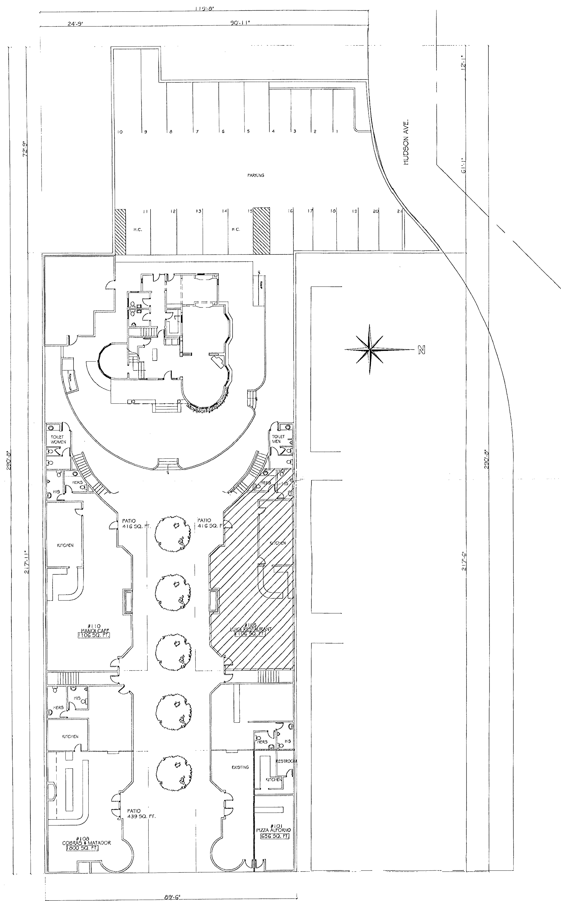
1 SITE PLAN 1/16"=1'
