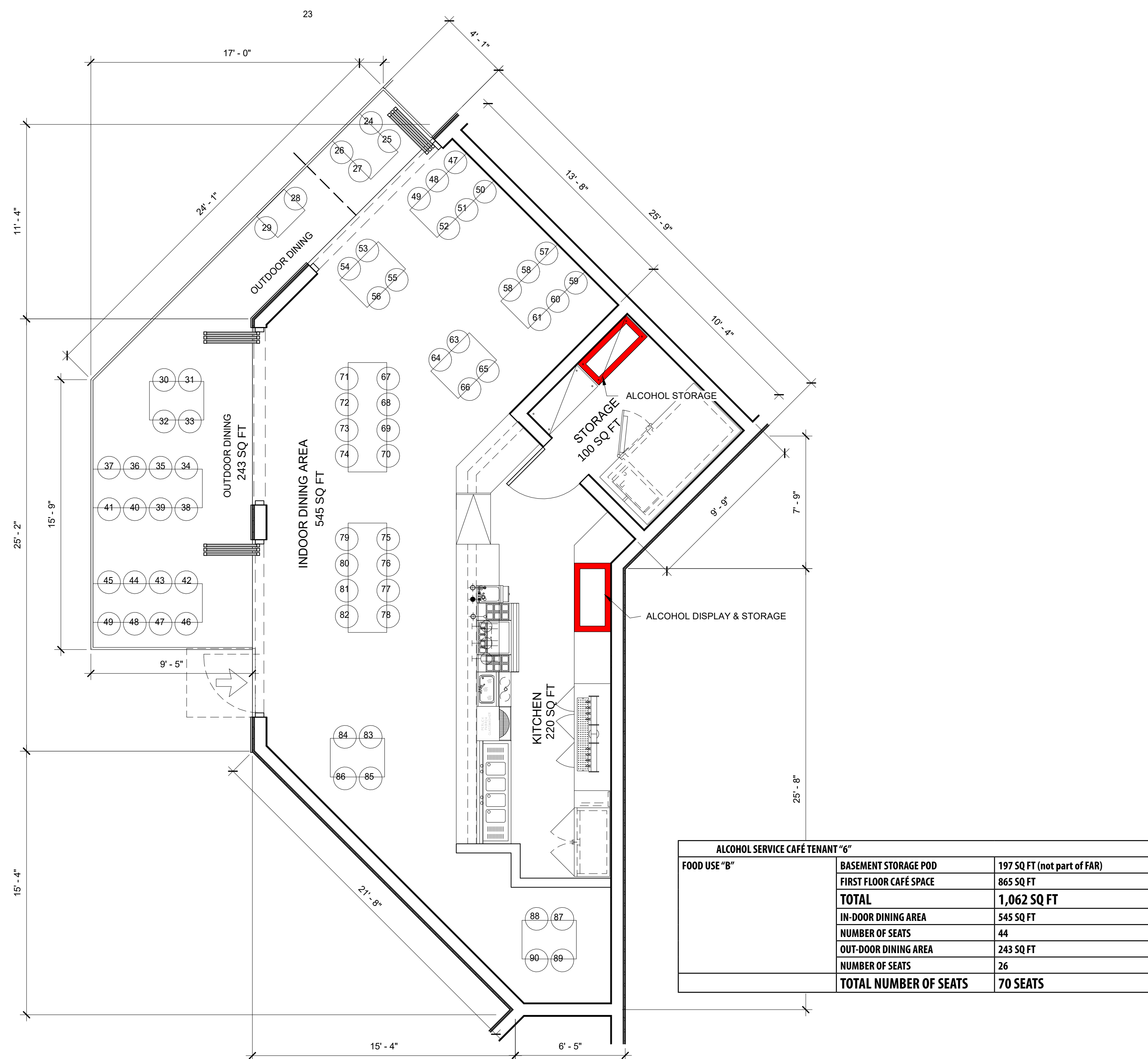
2 TENANT 6B 1/4" = 1'-0"
